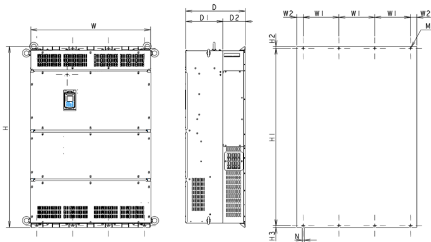
Abbildung 5 Externe Abmessungen des Umrichters (FRN500AR1S-4□ bis FRN710AR1S-4□)
