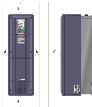
Abbildung 2.1 Montagerichtung und erforderliche Abstände
